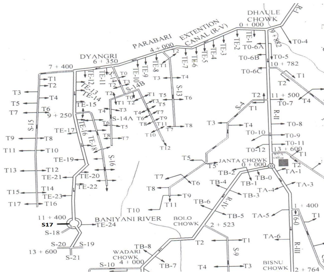
चित्र: S17 शाखा नहरको बिस्तारित कमाण्ड क्षेत्रफल
