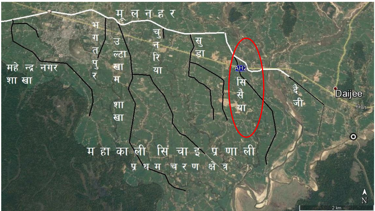
चित्र १ : महाकाली सिंचाइ प्रणाली प्रथम चरणको मूलनहर र सिसैया माइनर नहरको स्थिति नक्शा
