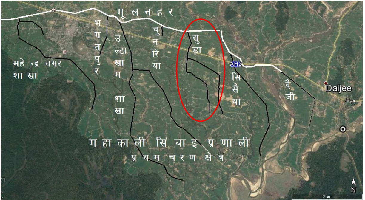
चित्र १ : महाकाली सिंचाइ प्रणाली प्रथम चरणको मूलनहर र सुडा माइनर नहरको स्थिति नक्शा
